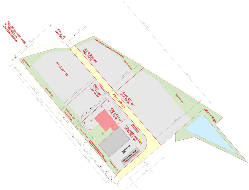
Lageplan Konzept
